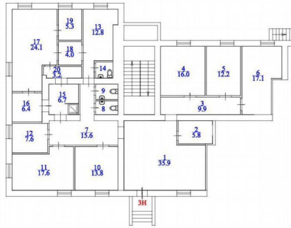
1-ый этаж
